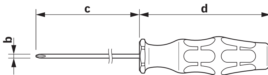
Esquema de dimensiones
