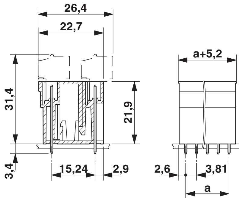
Maßzeichnung
