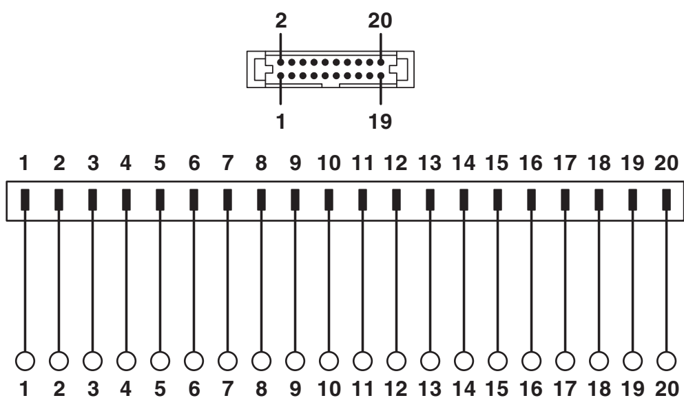
Schaltplan
