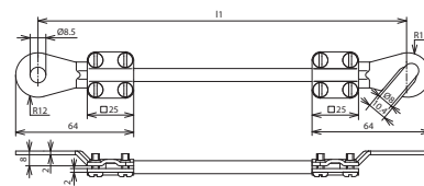
Maßbild EL10 L0.55M 1KSO 8.10 1KSG 8
