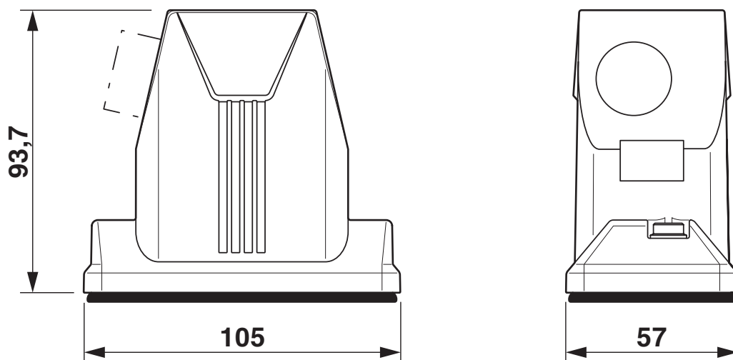
Maßzeichnung
