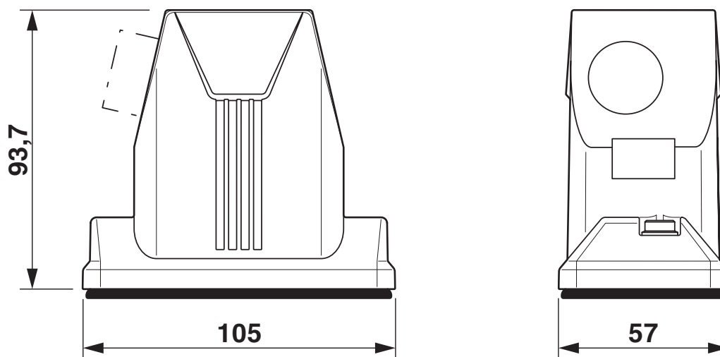
Dessin coté
