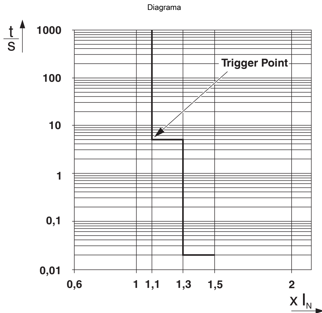
Curva característica de disparo 4 A
