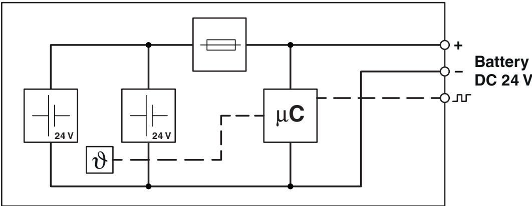
Blockschaltbild
