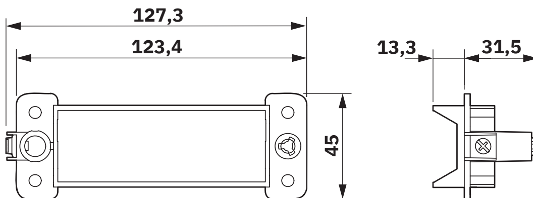
Dessin coté
