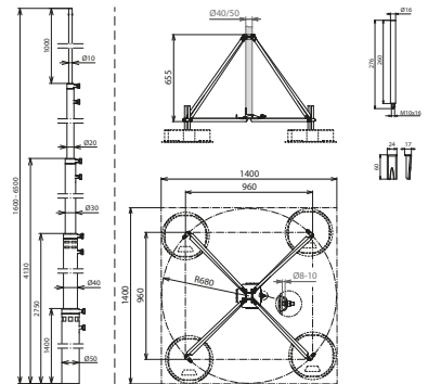
Maßbild FS T D50 1.6 6.5M AL VBS RA680
