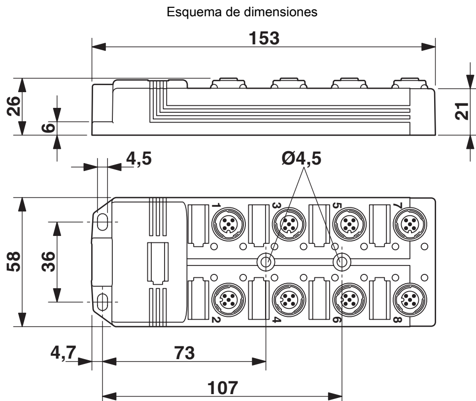
Plano esquemático
