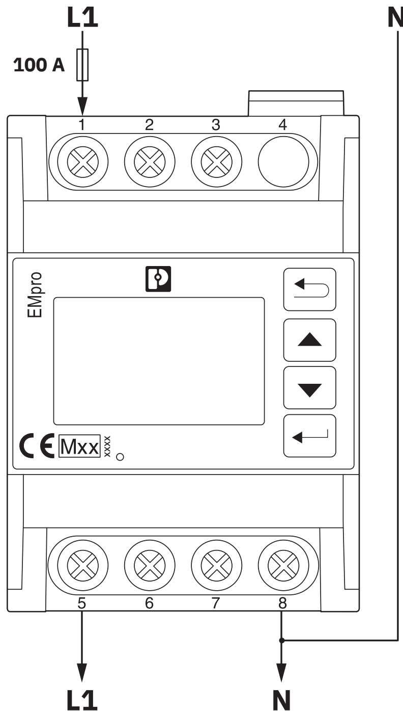
Dibujo de conexión
