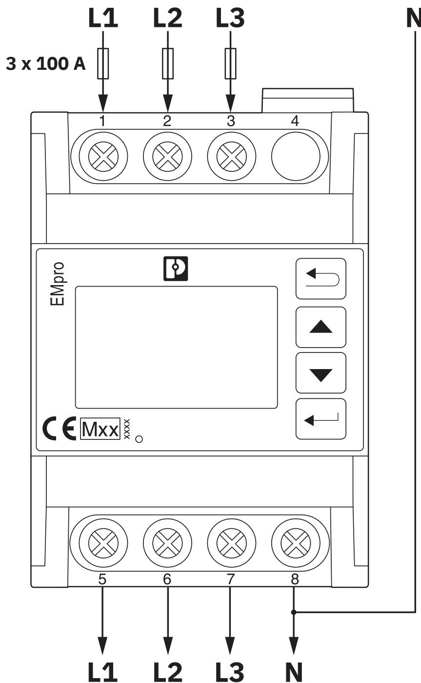
Dibujo de conexión
