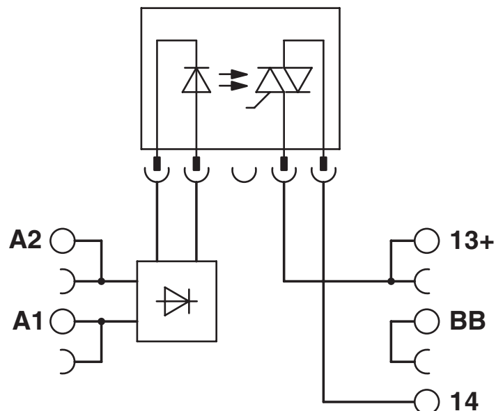
Diagrama eléctrico
