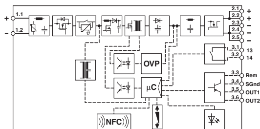
Blockschaltbild
