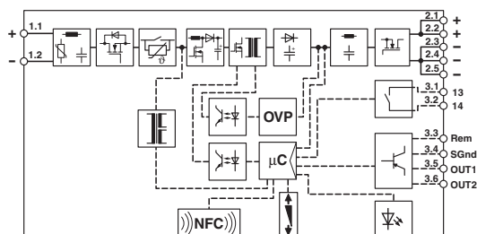
Schéma fonctionnel
