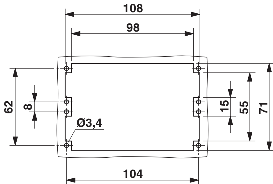
Montageausschnitt bei Verwendung ohne Gehäuse
