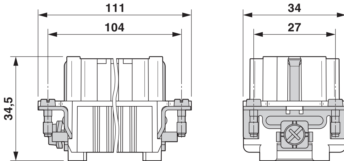
Maßzeichnung
