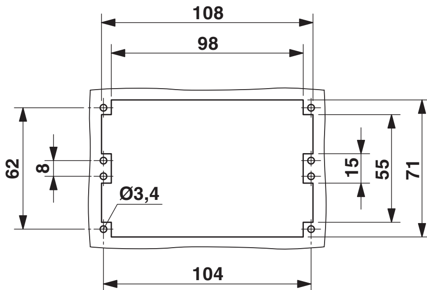
Sección de montaje en caso de uso sin caja
