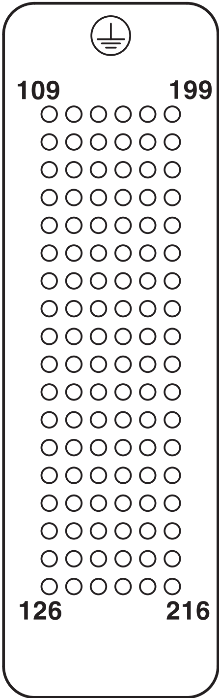
Plano esquemático
