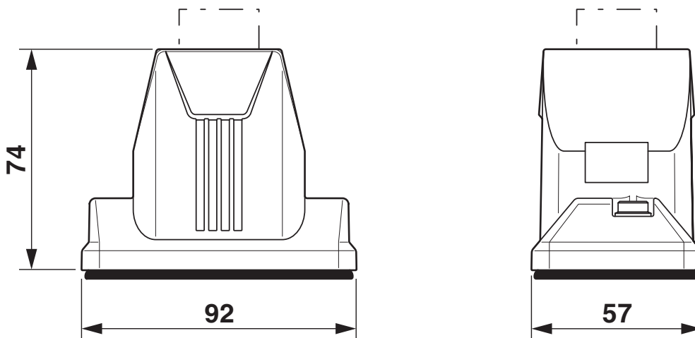
Maßzeichnung
