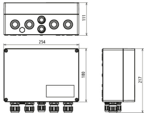
Dimensioni DCU 2 YPV 1100 2M 2S
