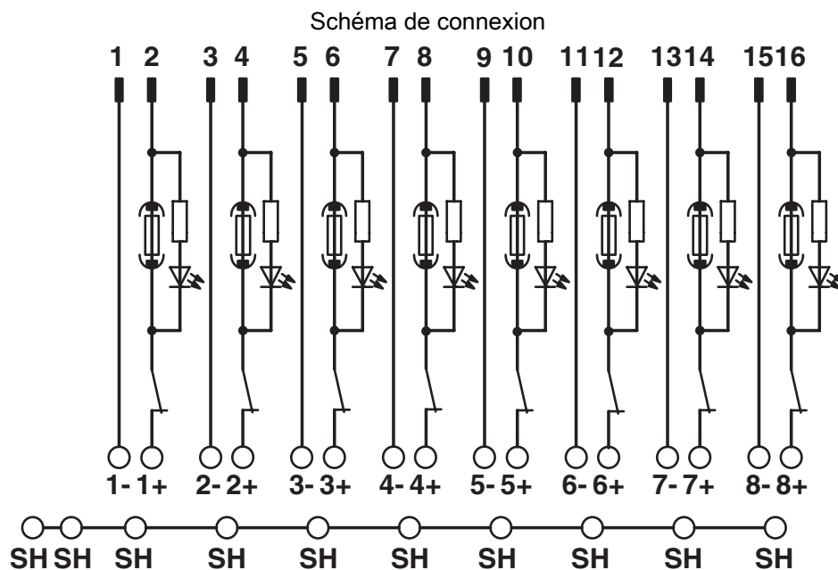
Schéma des connexions UM-DELTAV/A/SI/BFI/TP
