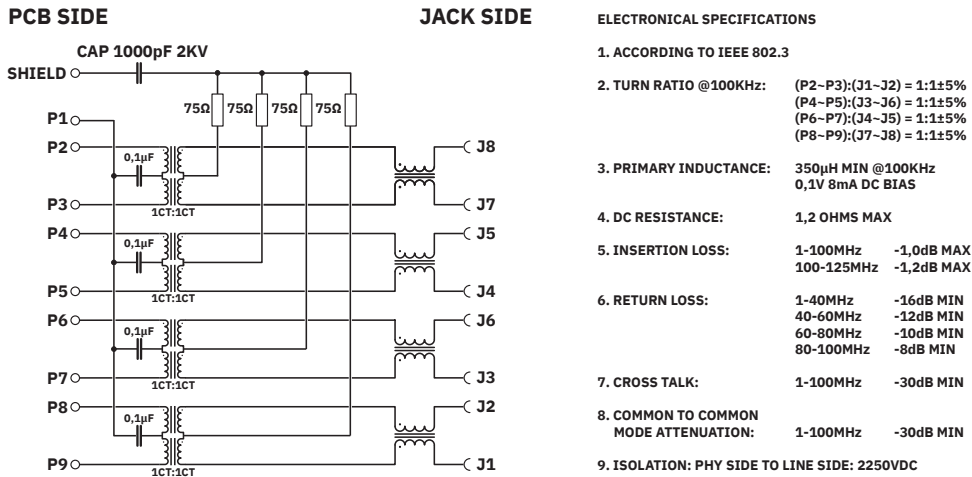
Diagrama eléctrico
