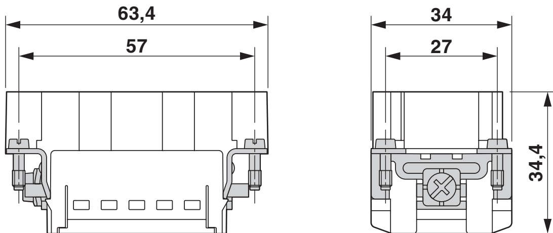
Maßzeichnung
