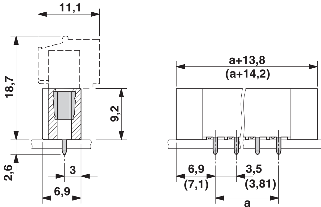
Dessin coté
