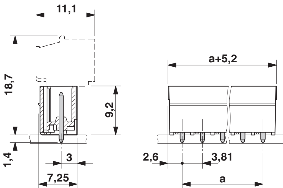
Dessin coté
