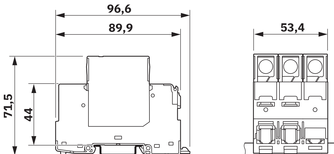
Maßzeichnung
