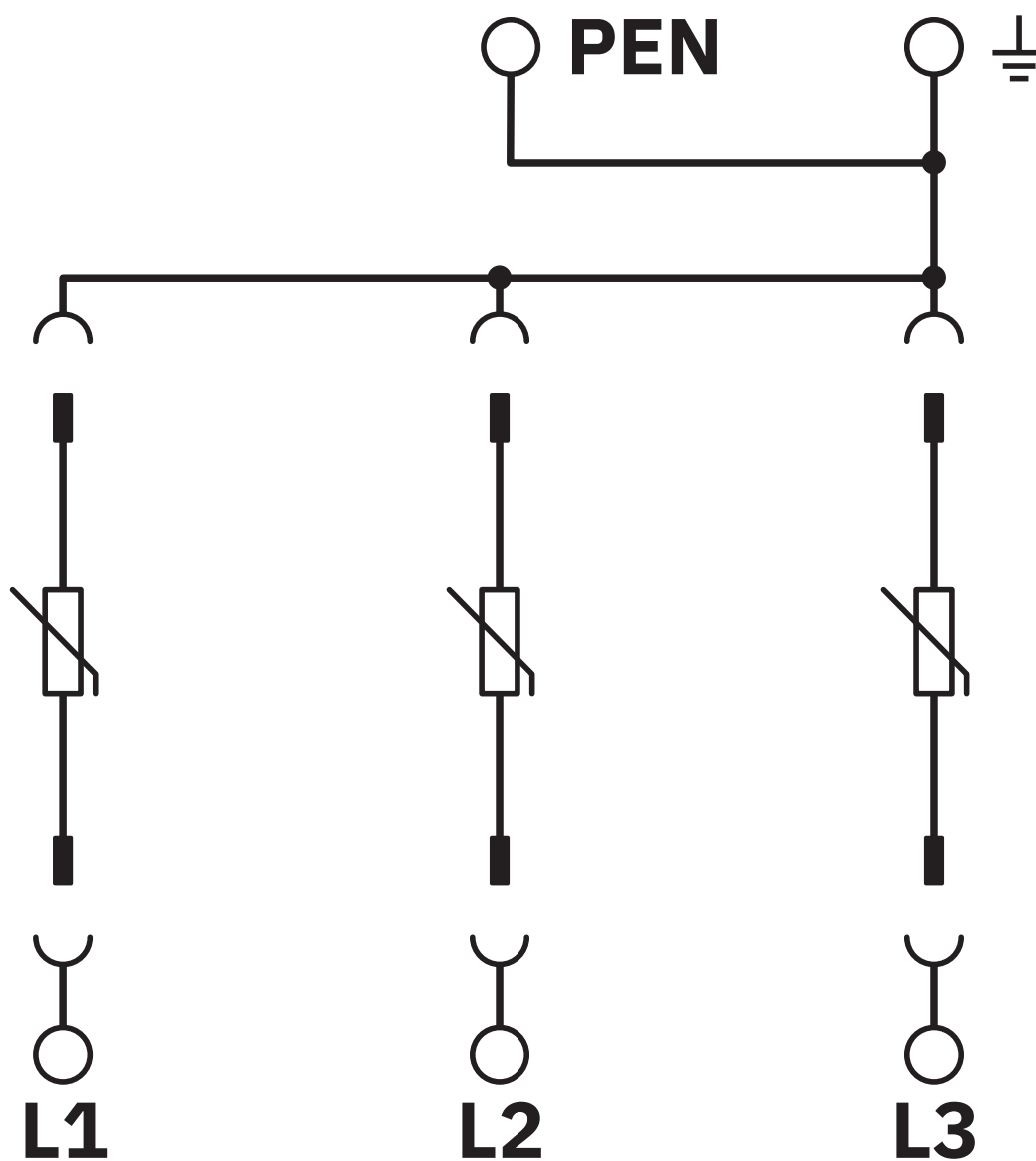
Diagrama eléctrico
