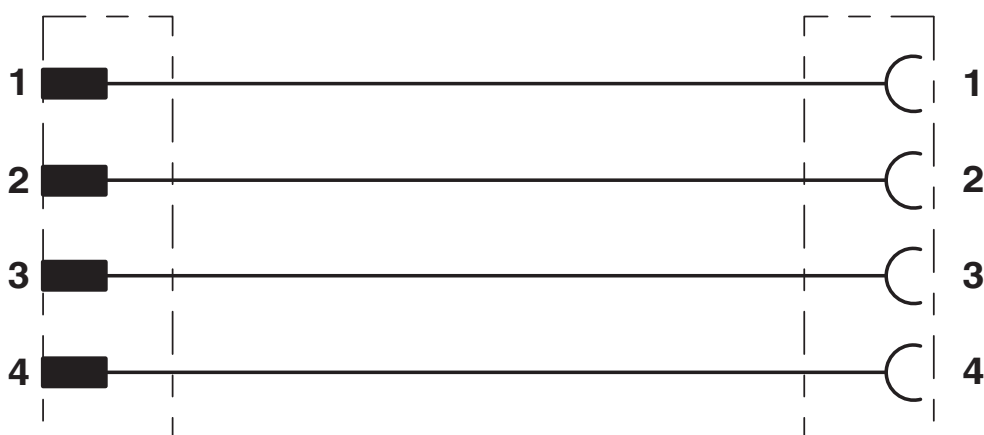
Diagrama eléctrico
