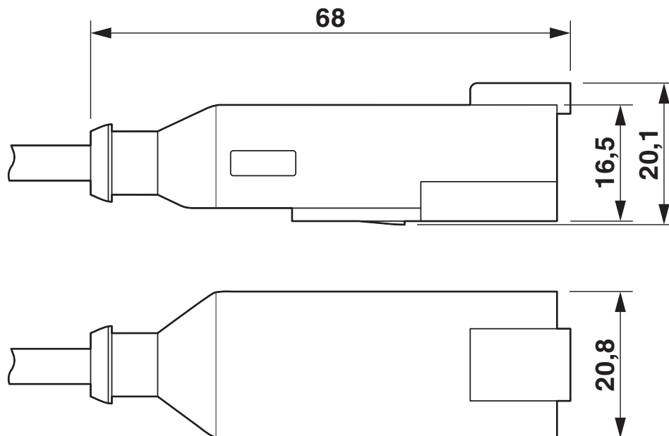
DEUTSCH DT04-4P, vue de dessus et vue de côté
