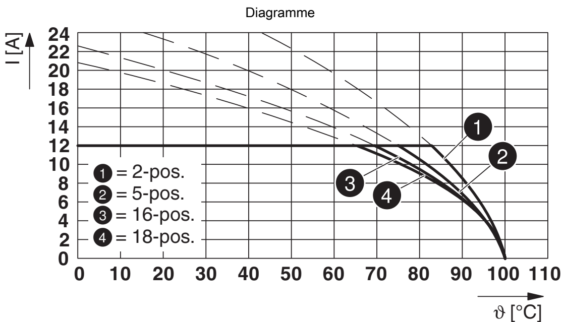
Type : FKCV(W/R) 2,5/...-ST avec MSTBW 2,5/...-G
