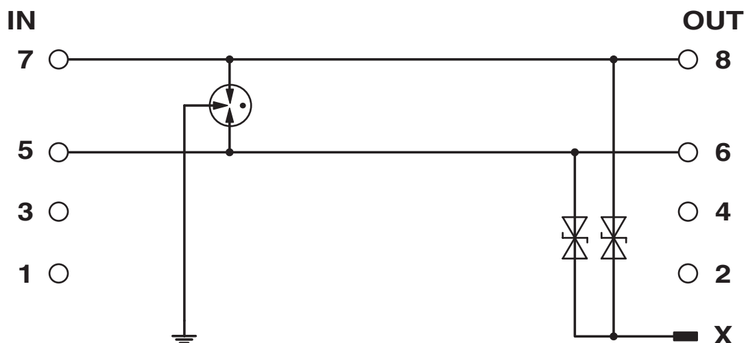
Schaltplan
