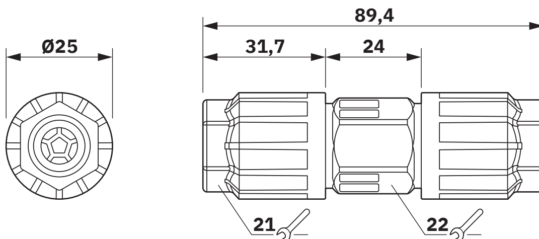
Dessin coté
