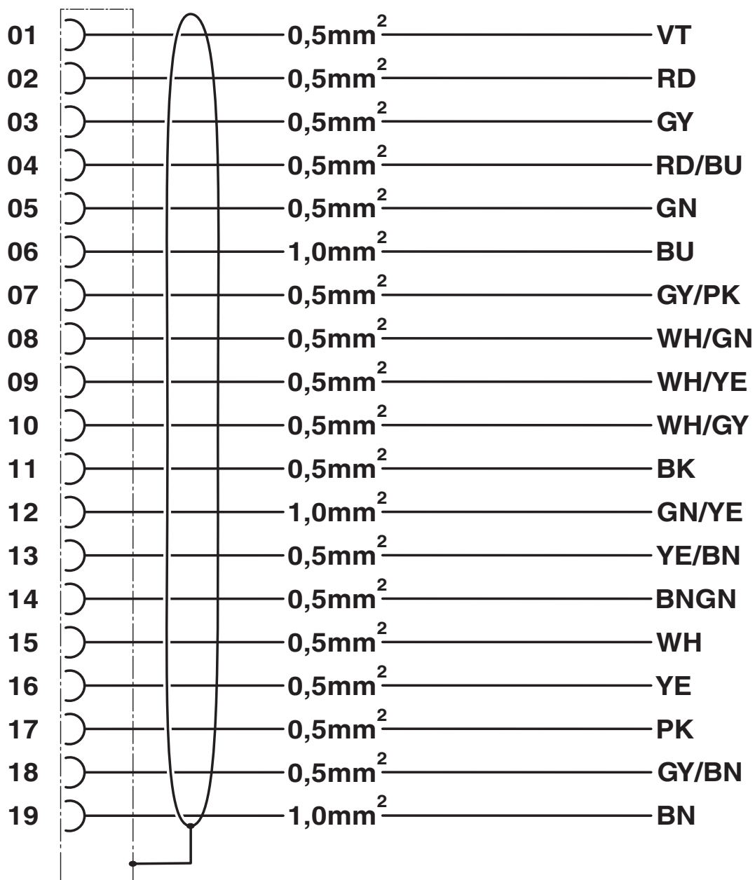
Diagrama eléctrico
