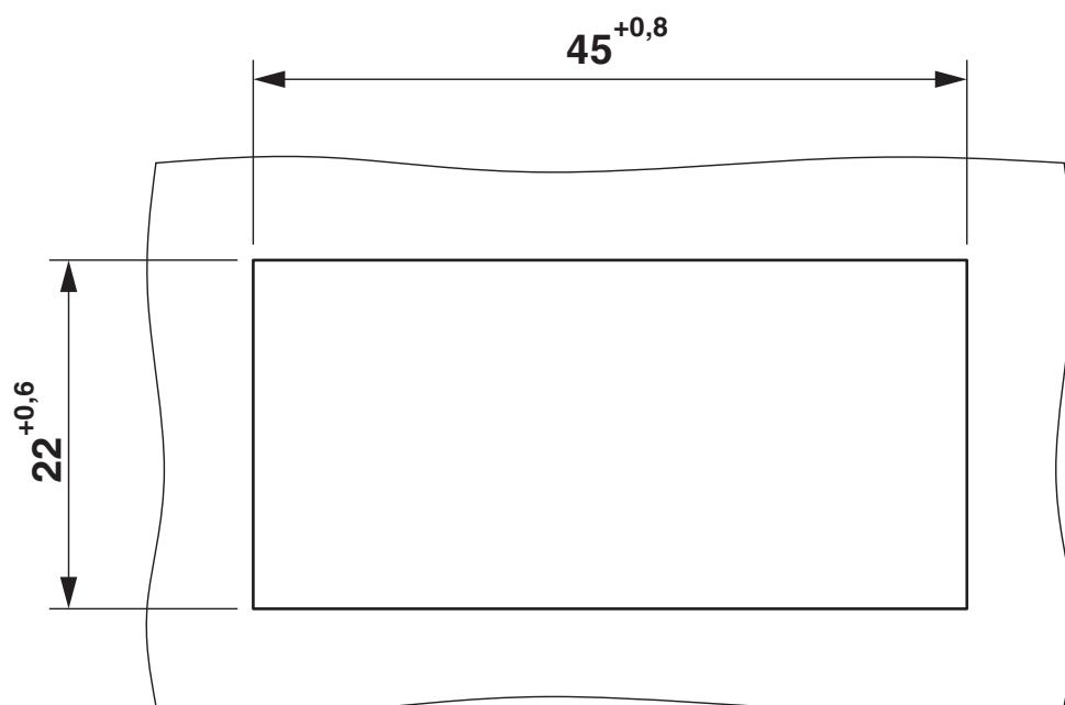
Dessin coté
