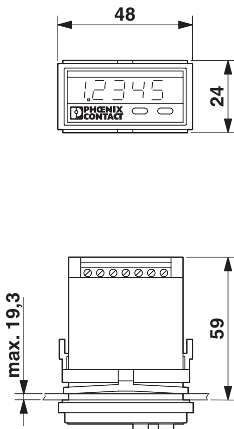
Dessin coté
