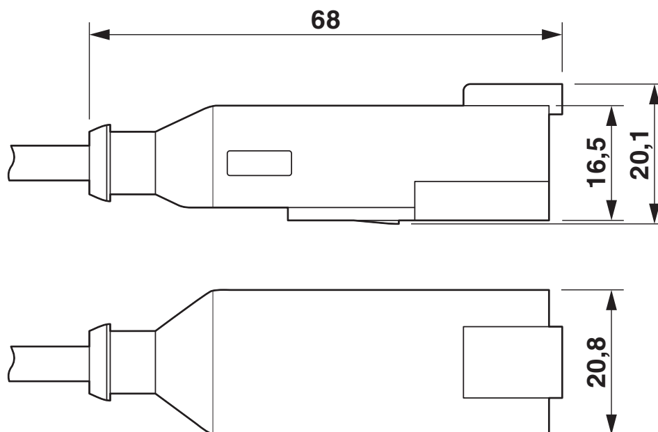
Dessin coté
