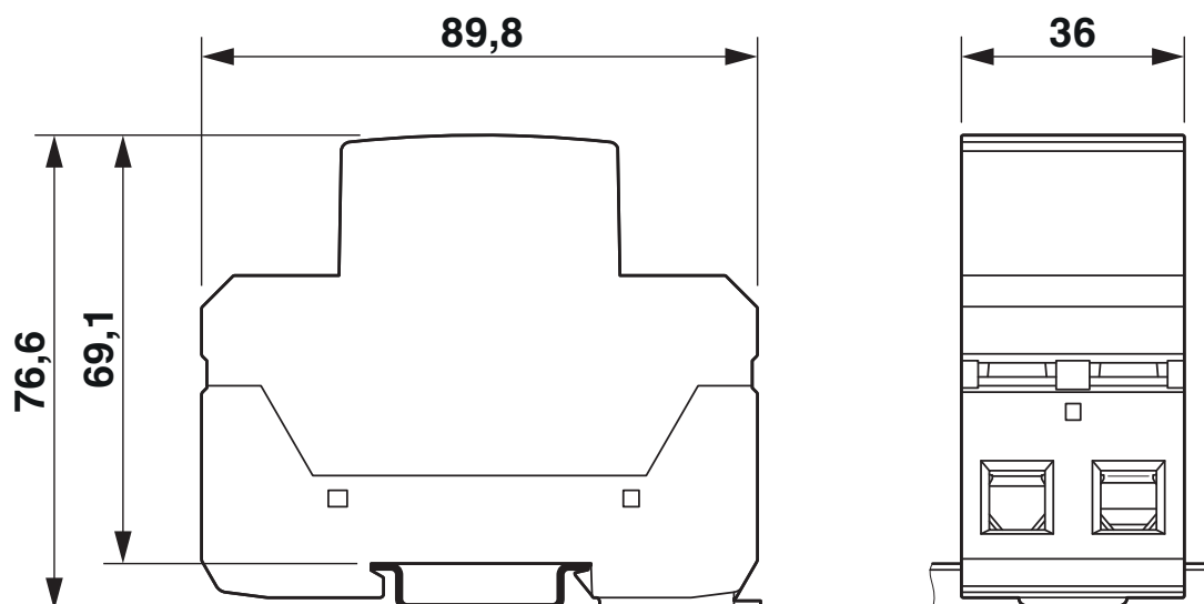
Maßzeichnung
