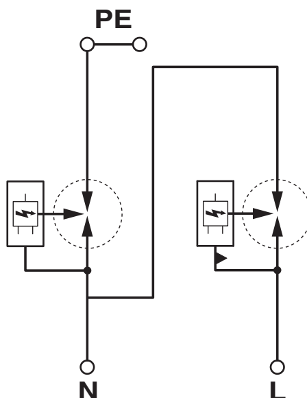
Diagrama eléctrico
