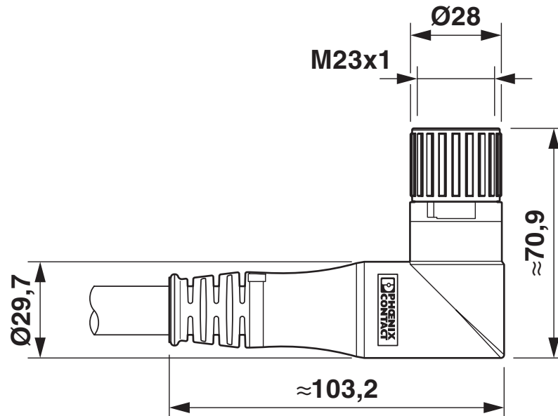
Maßzeichnung
