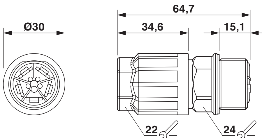
Maßzeichnung
