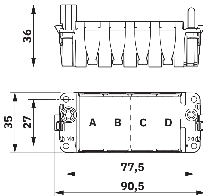
Dessin coté
