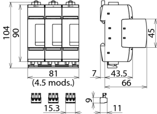
Dimensiones del DG ME YPV SCI 1500 FM
