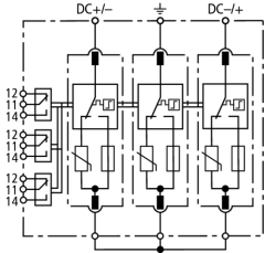
Esquema del DG ME YPV SCI 1500 FM
