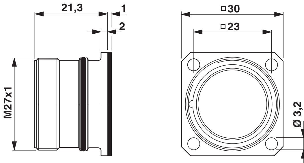
Maßzeichnung
