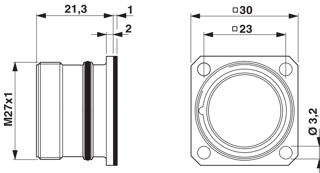
Dessin coté
