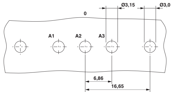
Esquema de taladros/geometría pads soldadura
