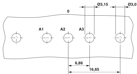
Gabarit perçage / géom. pastille soudage
