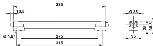
Maßzeichnung
