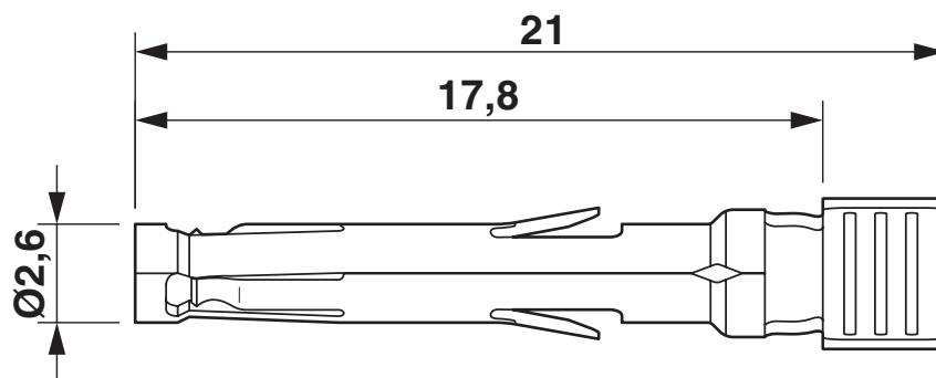
Maßzeichnung
