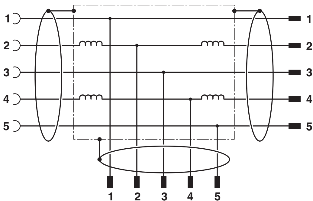
Ocupación de contactos del conector macho M12 y del conector hembra M12
