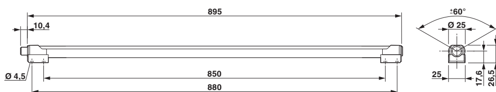
Dessin coté
