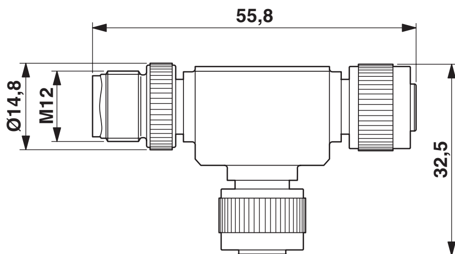
Dessin coté
