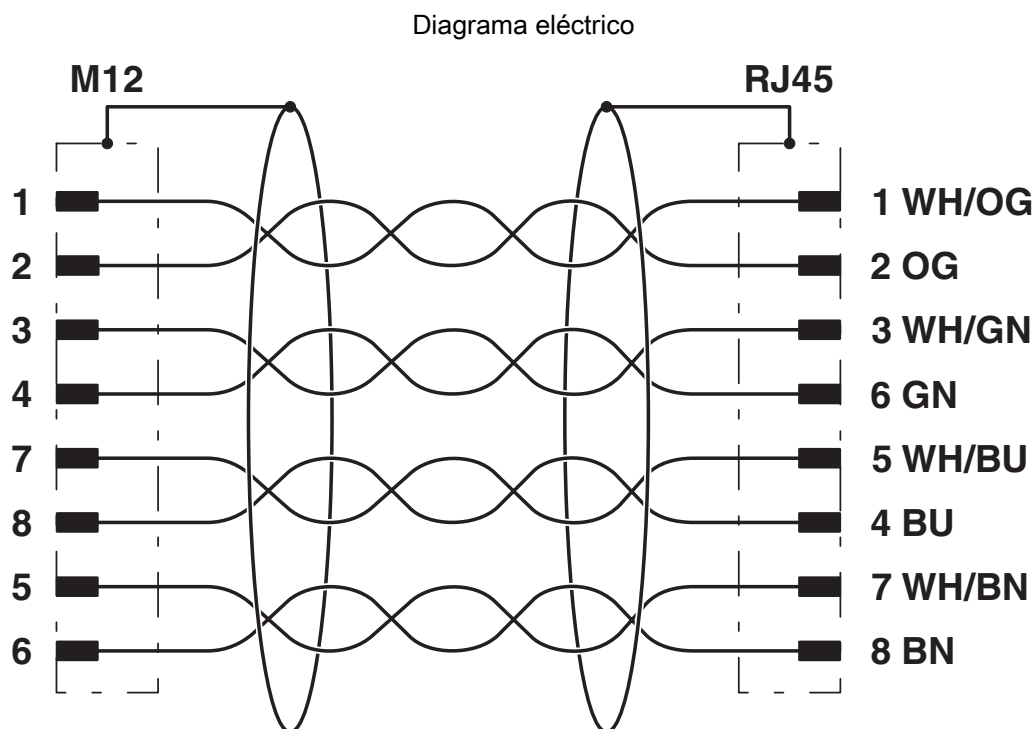
Ocupación de contactos de los conectores macho M12 y RJ45
